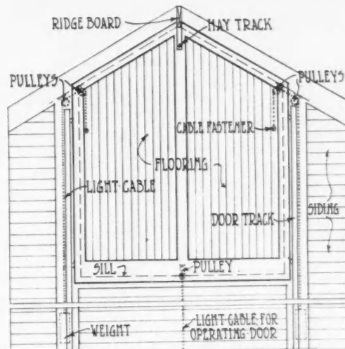
ELEVATION OF HAY MOW DOOR
