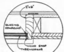
JAMB SECTION-C-C
