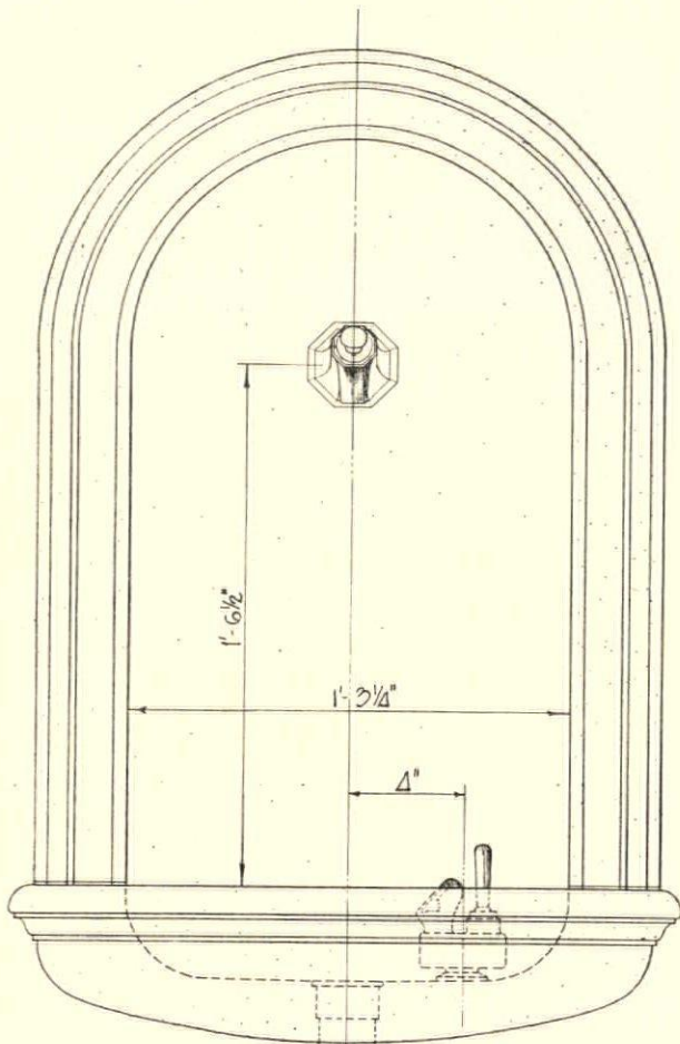
· ELEVATION ·
