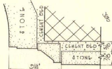
· TRIM · DETAIL ·
